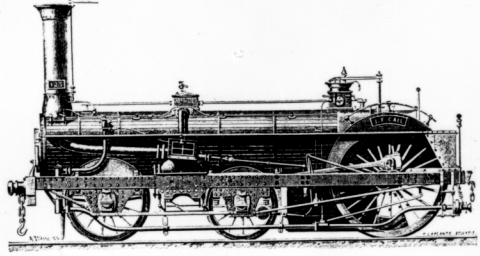
-Máquina de gran velocidad; tipo Crampton
